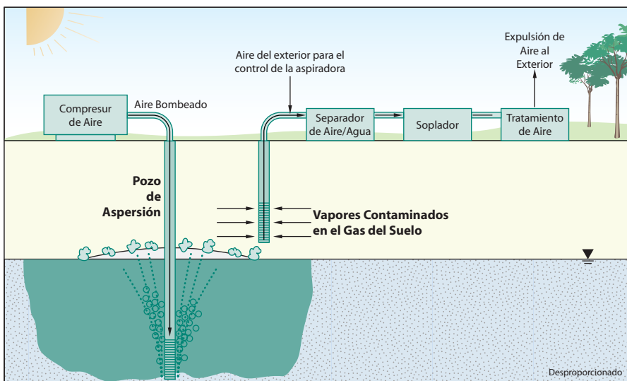
Figura 1- Sistema de la Aspersión de Aire
