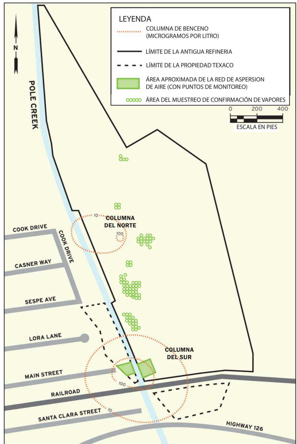
Figura 2: Ubicación del Muestreo de Vapores y Red de Aspersión de Aire (aspersión de aire solo on la columna del sur)
